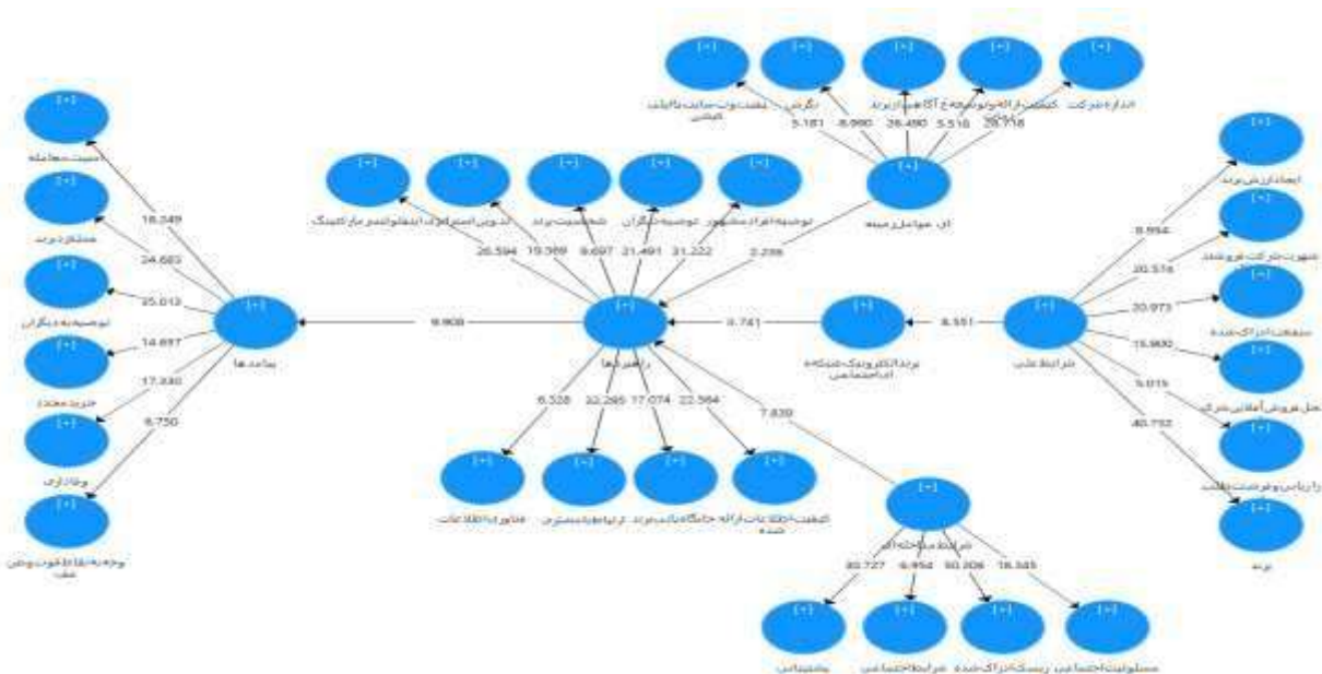
شکل ۷: خروجی مدل درونی (معادلات ساختاری) مدل پژوهش در نرم افزار smart pls
