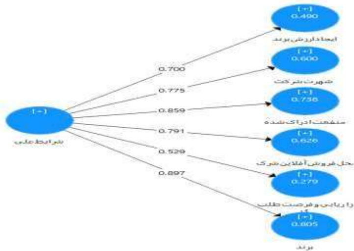
شکل ۱: خروجی مدل اندازه گیری شرایط علی
