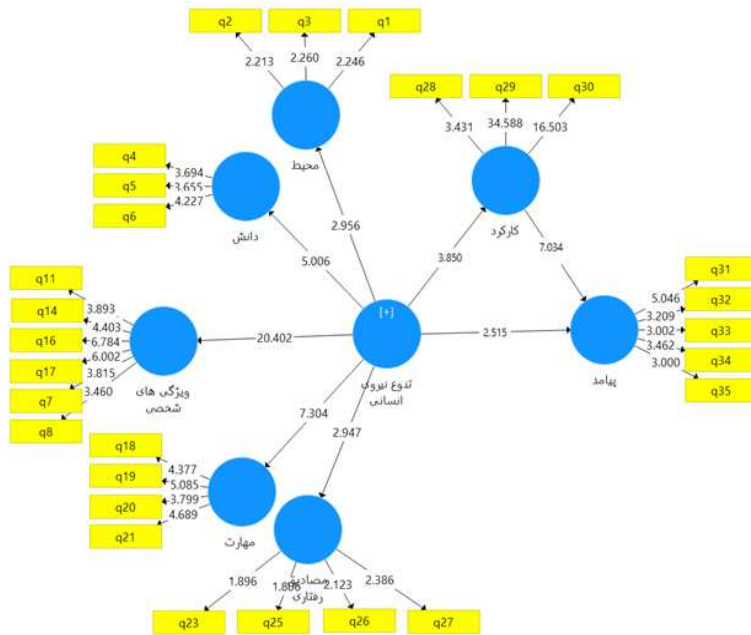
شکل ۶- اجرای مدل اصلاح شده
