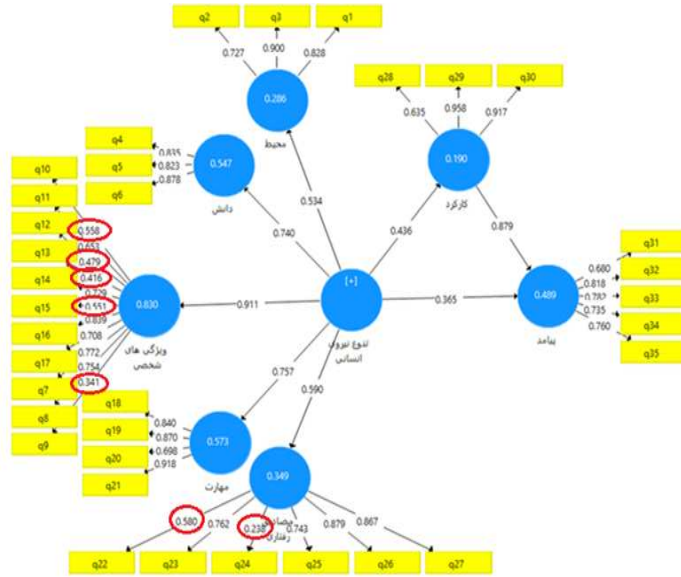
شکل ۵- اجرای مدل پیش از آزمون همگنی و شناسایی بارهای عاملی قابل حذف
