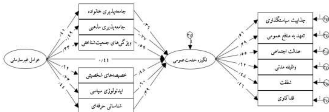
شکل ۳. نتایج معادلات ساختاری برای بررسی مدل تاثیر متغیر
